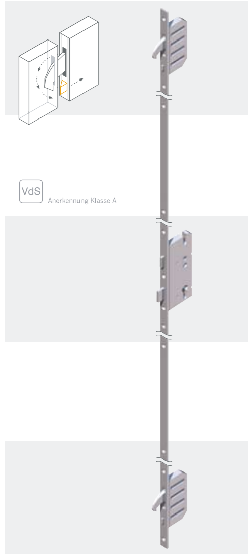
autoLock AV2 – zamek z ryglowaniem automatycznym
