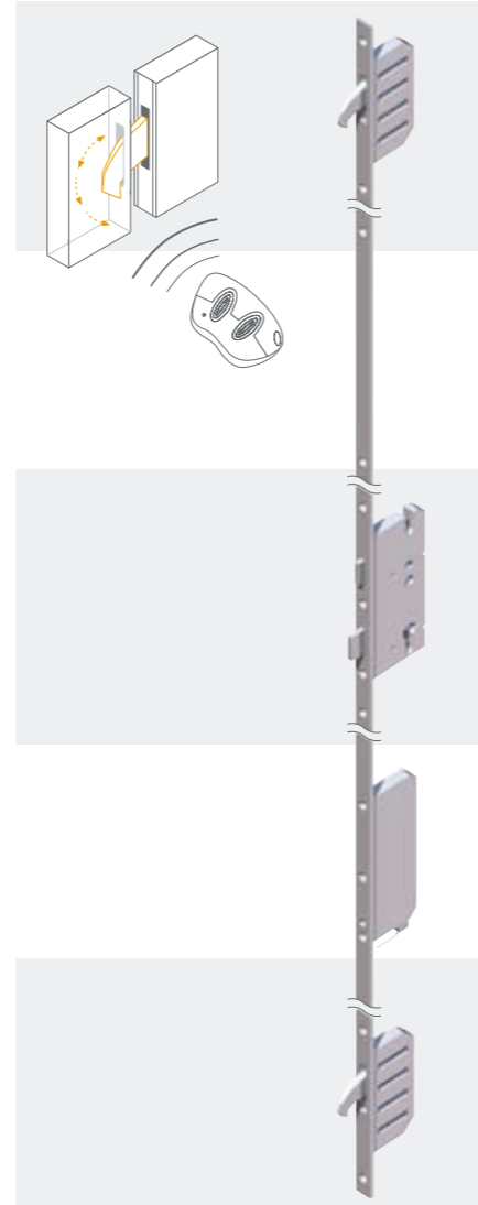
blueMotion – zamek z napędem elektrycznym w skrzydle
